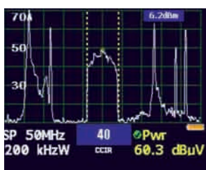
ANALIZADOR DE ESPECTRO EN MODO ÓPTICO
